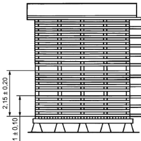
Рисунок А.9 - Горизонтальные каналы в рядовом штабеле
