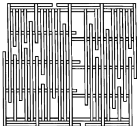
а) Укладка в глубокий потай
