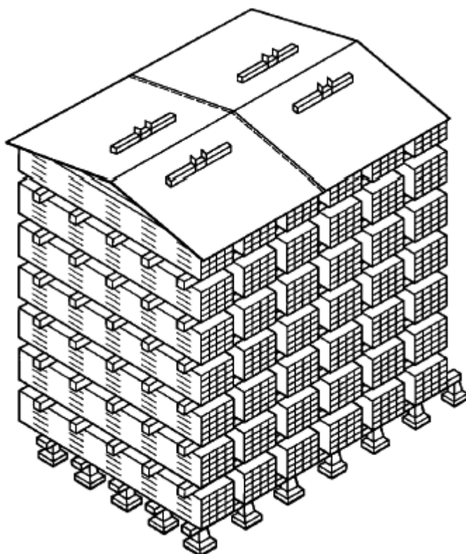
Рисунок А.6 - Пакетный штабель
