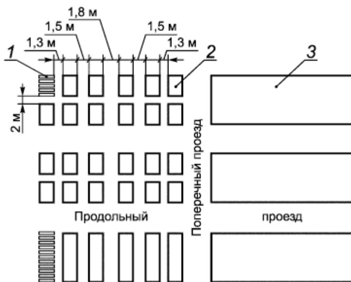
Рисунок А.1 - Планировка групп рядовых штабелей
