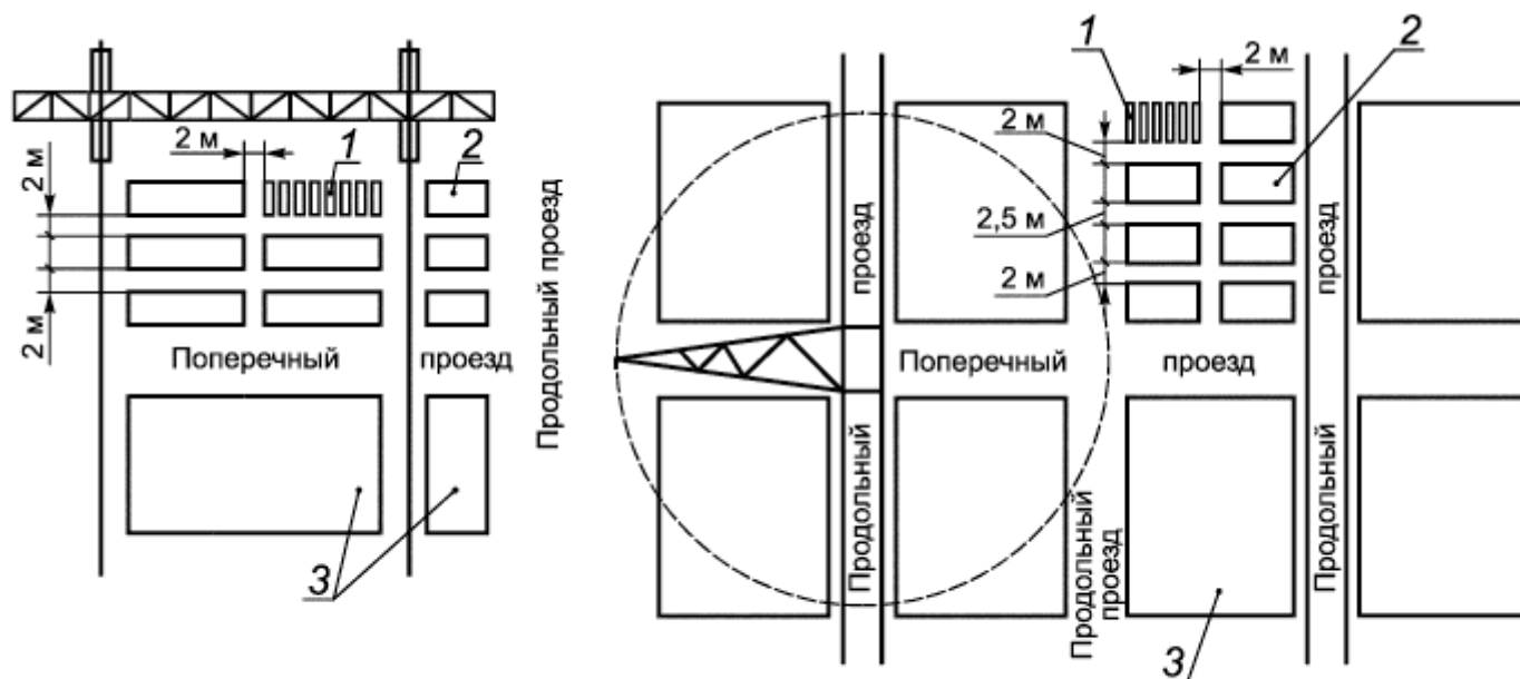
а) Укладка козловым краном
