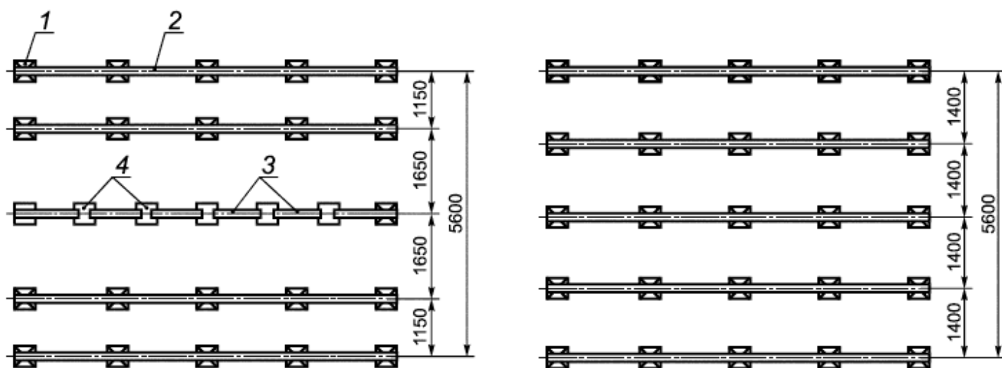
а) Укладка автопогрузчиком
