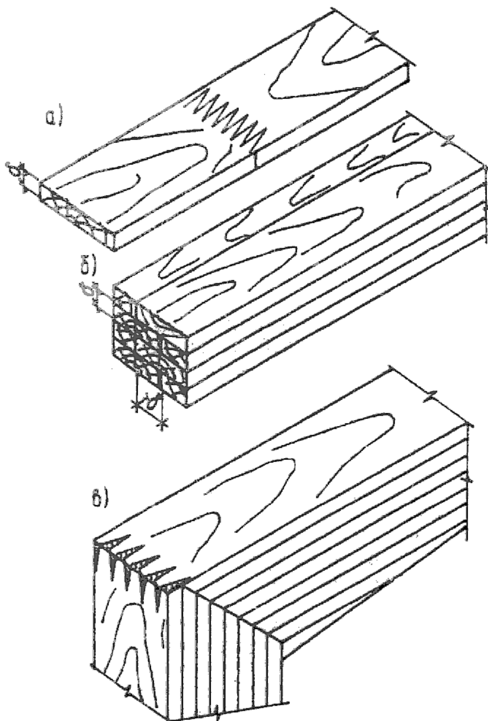
Рис. 6 Клеевые соединения
