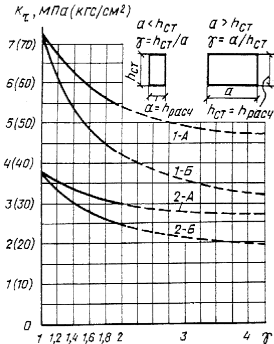
Рис. 3. Графики для определения k_{\tau}
