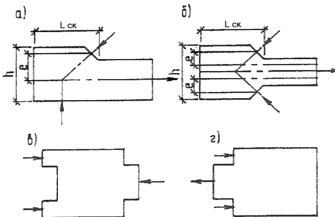
Рис. 5. Врезки в элементах соединений
