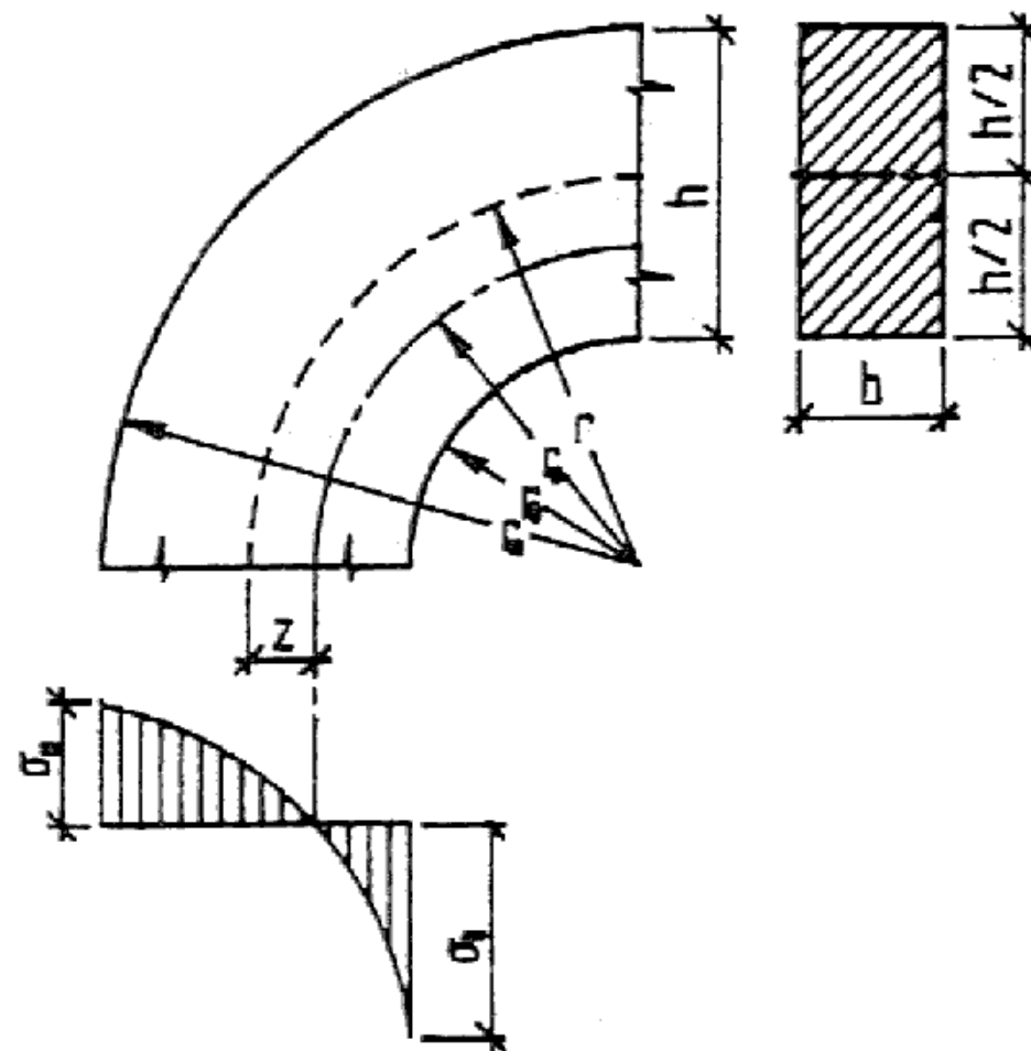
Рис. 16. Расчетная схема к определению напряжений в криволинейной части гнутоклееных рам
