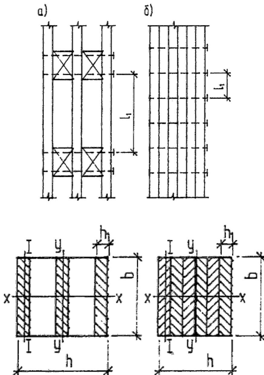
Рис. 2. Составные элементы
